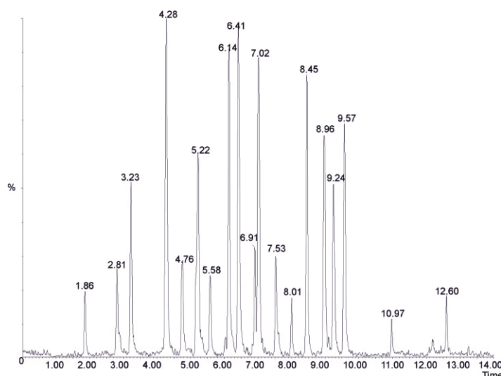
Separace analytů s využitím ultračinné kapalinové chromatografie a hmotnostně-spektrometrické detekce s fotoionizací za atmosférického tlaku.
